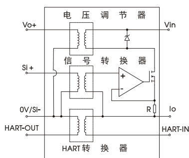
图 2 功能原理框图
